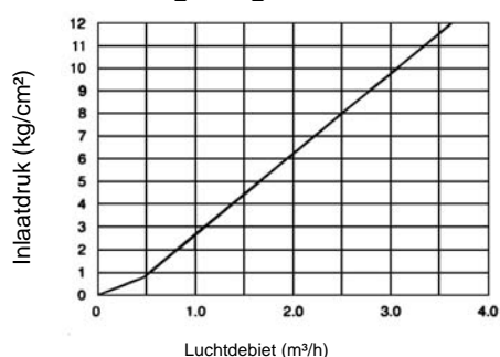
Automatische ontluchter 1", 2" (A)
