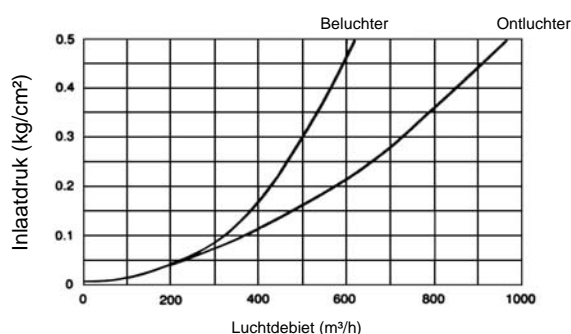
Automatische ont- en beluchter 2" (K, A)
