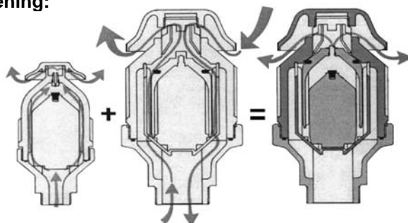
Automatische ontluchter 1", 2" (A)
