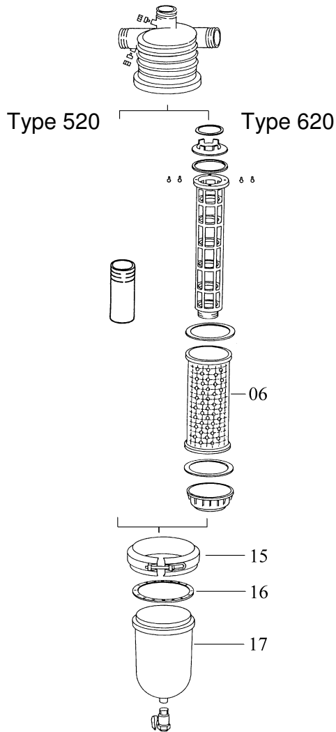
2" Zandafscheider
