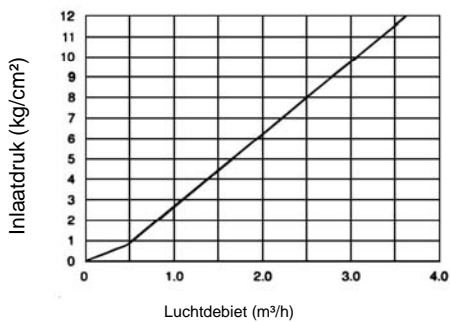
Automatische ontlufter 1", 2" (A)
