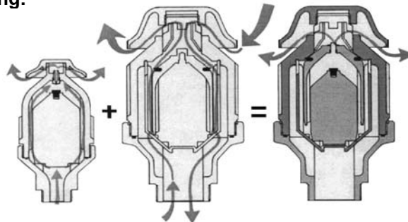
Automatische ontlufter 1", 2" (A)
