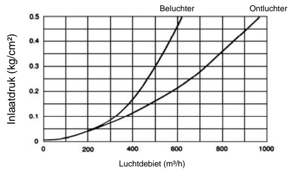
Automatische ont- en beluchter 2" (K, A)
